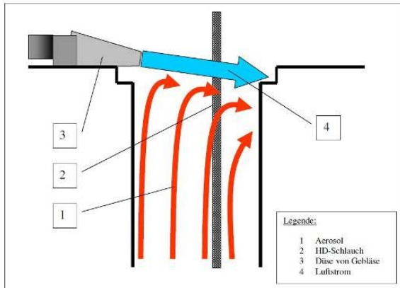
Beispiel: Kanalreinigung mit HDS-Fahrzeugen – Luftschleierabspernung (Quelle: TRBA 220, WSW)
