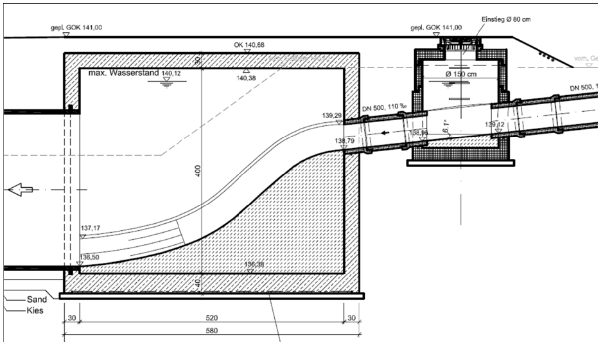
Beispiel: Gestaltung Absturzbauwerk (Quelle: DAR)
